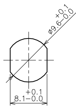
取付穴寸法
