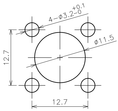
取付穴寸法
