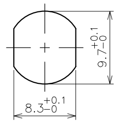
パネル取付穴寸法
