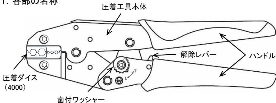
図1 圧着工具各部の名称
