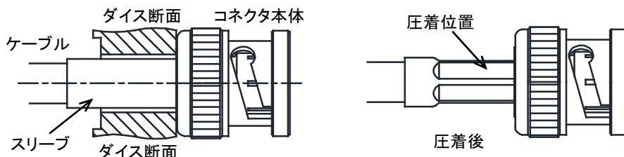
図4 スリーブの圧着
