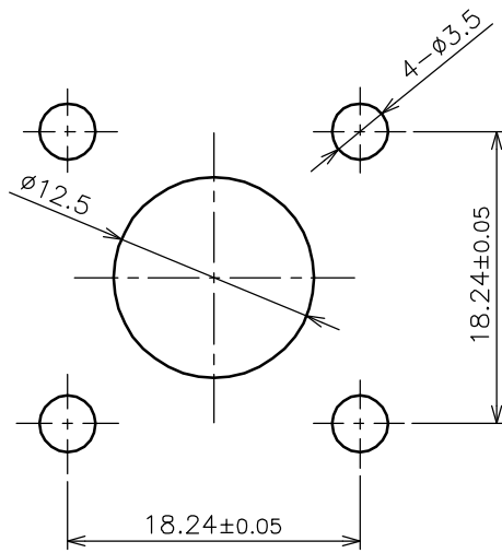
取り付け穴参考図
