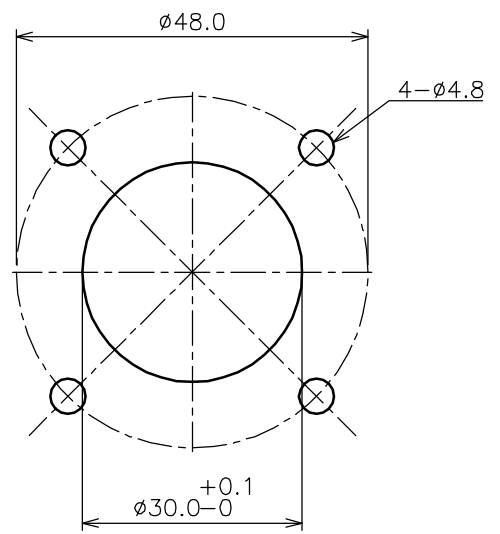
取付穴寸法
