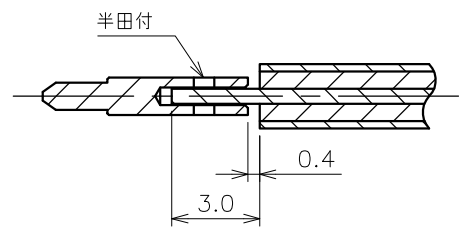
端末加工寸法
