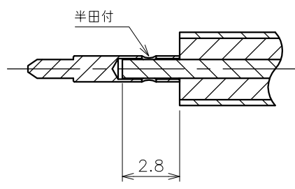
端末加工寸法
