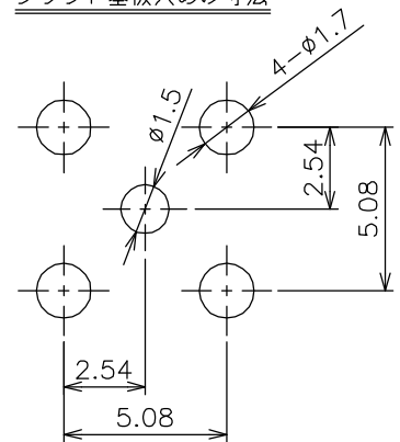
プリント基板穴あけ寸法
